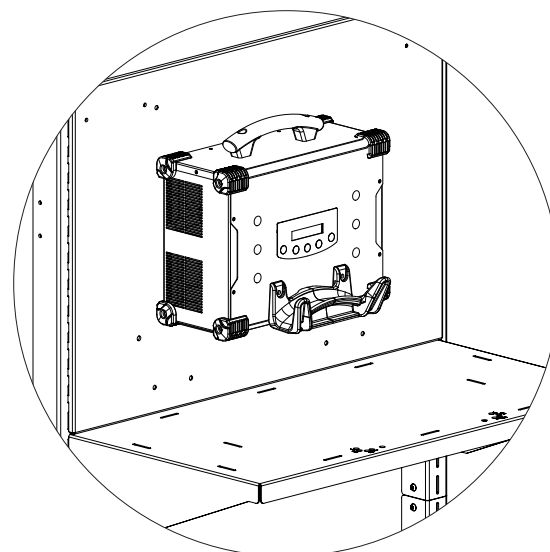
Вертикальный Gysflash
