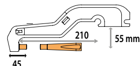
C2 - 8bar/550 daN
